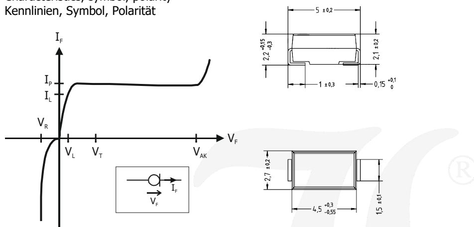
Dimensions - Maße [mm]
